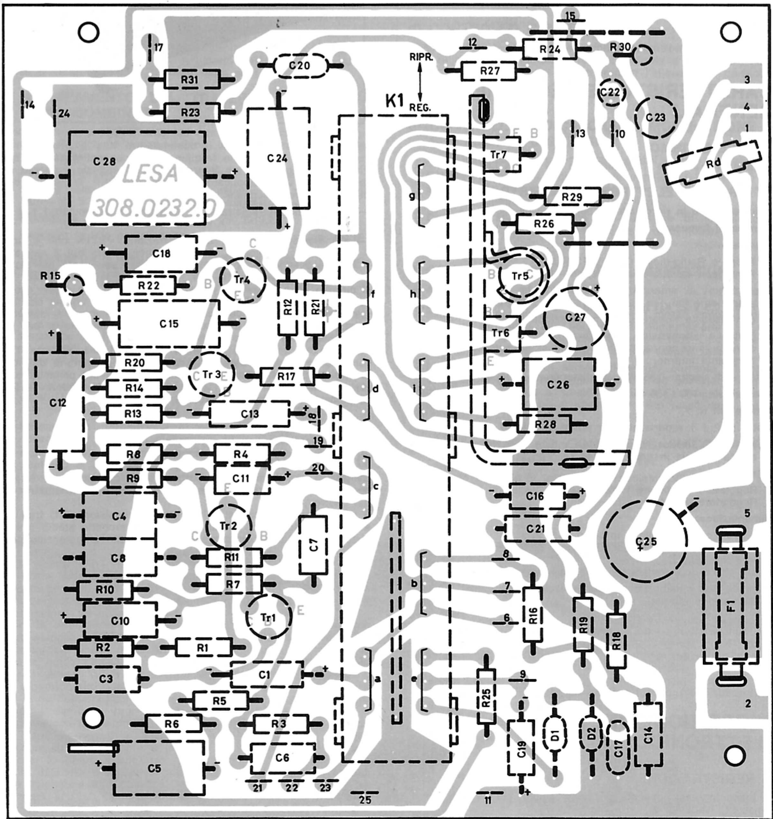
FIG. 8 - Circuito stampato amplificatore Renas CM 22
